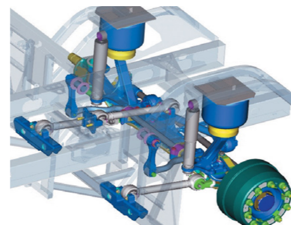
Передняя пневматическая подвеска
