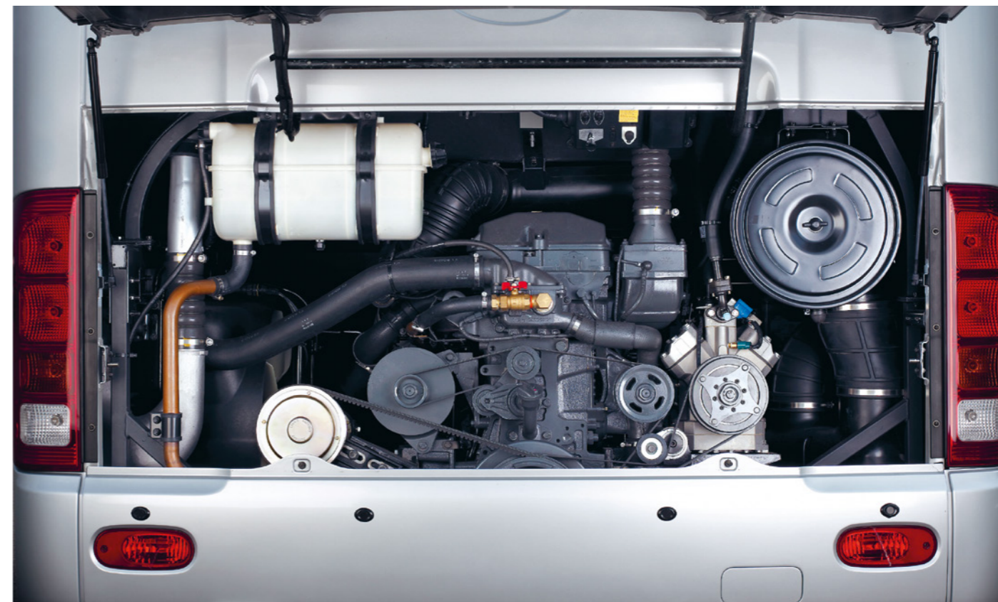
Легкий доступ к основным узлам двигателя
