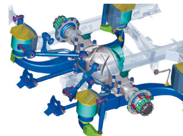
Задняя пневматическая подвеска
